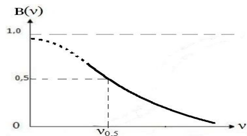
Рис. 1. Вероятностная модель (тренд) зависимости вероятностей успешного целераспределения B(\nu)
