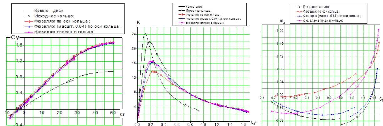
Рис. 14. Влияние положения и размеров фюзеляжа. Результат панельно-вихревого метода
