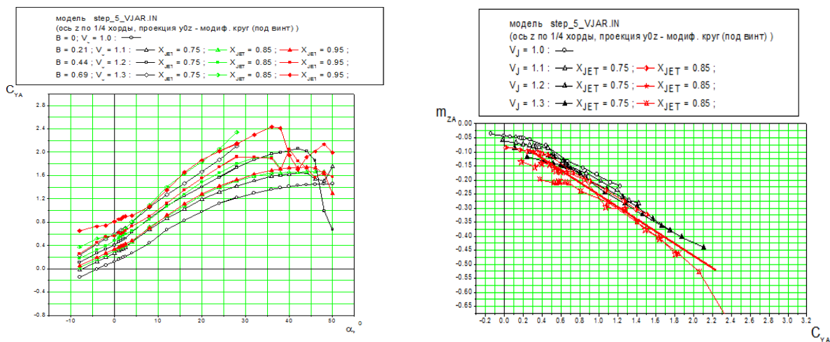
Рис. 12. Влияние струи работающего винта. Результат панельно-вихревого метода
