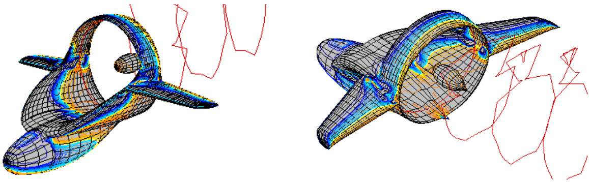
Рис. 9. Результирующая компоновка без ГО
