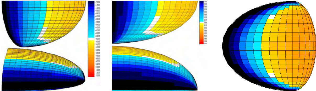
Рис. 3. Расчетные модели крыльев малого удлинения одинакового размаха
