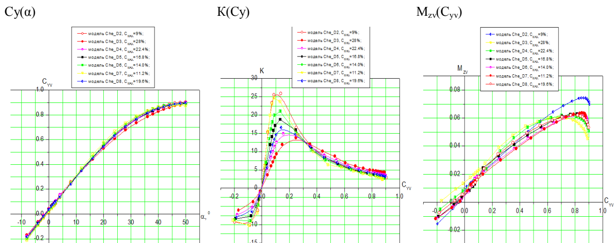
Рис. 11. Влияние формы крыла. Результат панельно-вихревого метода
