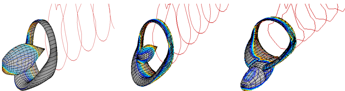
Рис. 8. Расчетные модели для исследования влияния фюзеляжа
