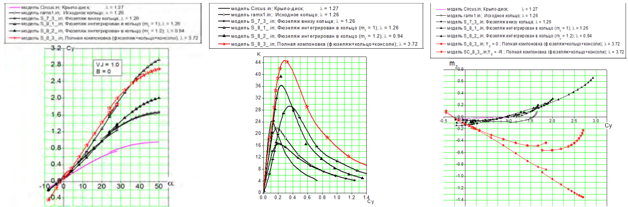
Рис. 15. Влияние компоновочных решений. Результат панельно-вихревого метода
