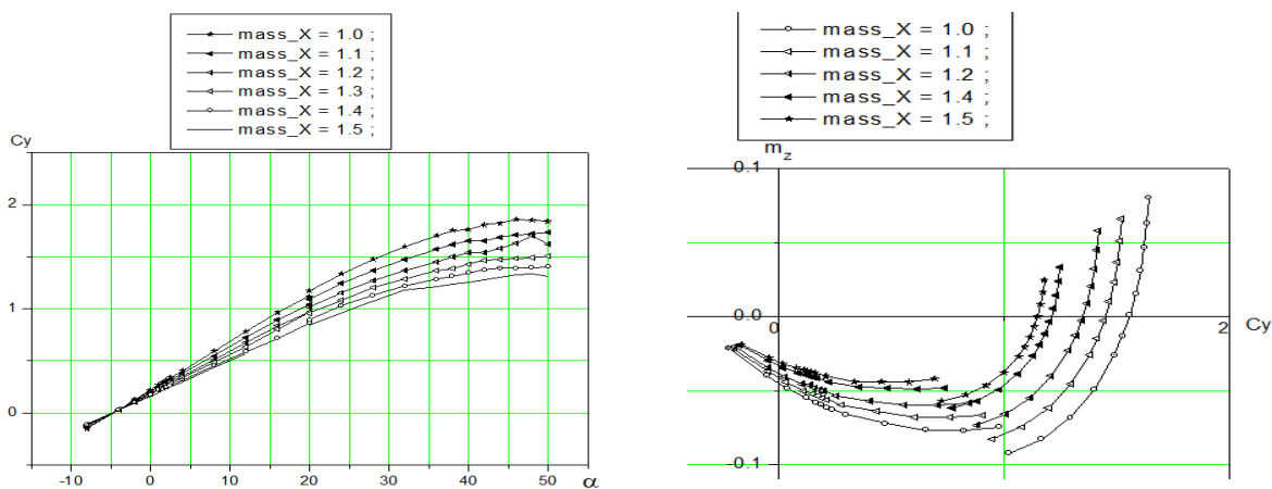
Рис. 13. Влияние масштаба кольца по оси x. Результат панельно-вихревого метода
