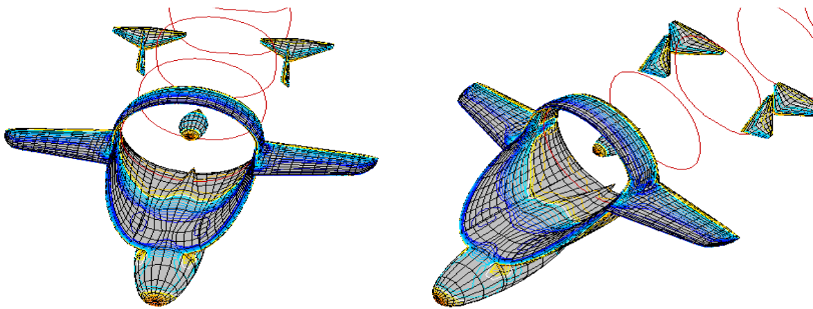
Рис. 10. Результирующая компоновка с ГО
