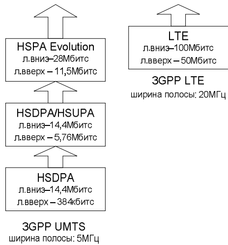
Рис. 2. Последовательное развитие технологий передачи данных
