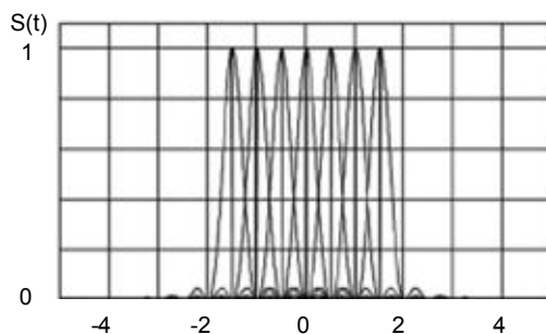
Рис. 4. Энергетический спектр сигнала OFDM
