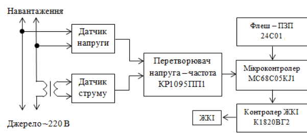
Рис. 2. Структурна схема найпростішого лічильника електроенергії
