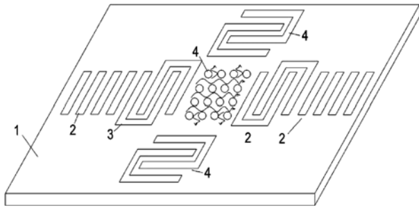
Рис. 1. Структура гіроскопа на поверхневих акустичних хвилях:
