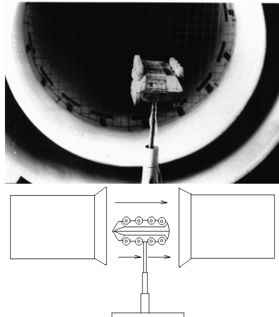
Рис. 3. Модель ЛБПМ в аеродинамічній трубі
