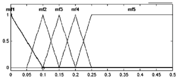
Рис. 6. Функции принадлежности для коэффициента проскальзывания
