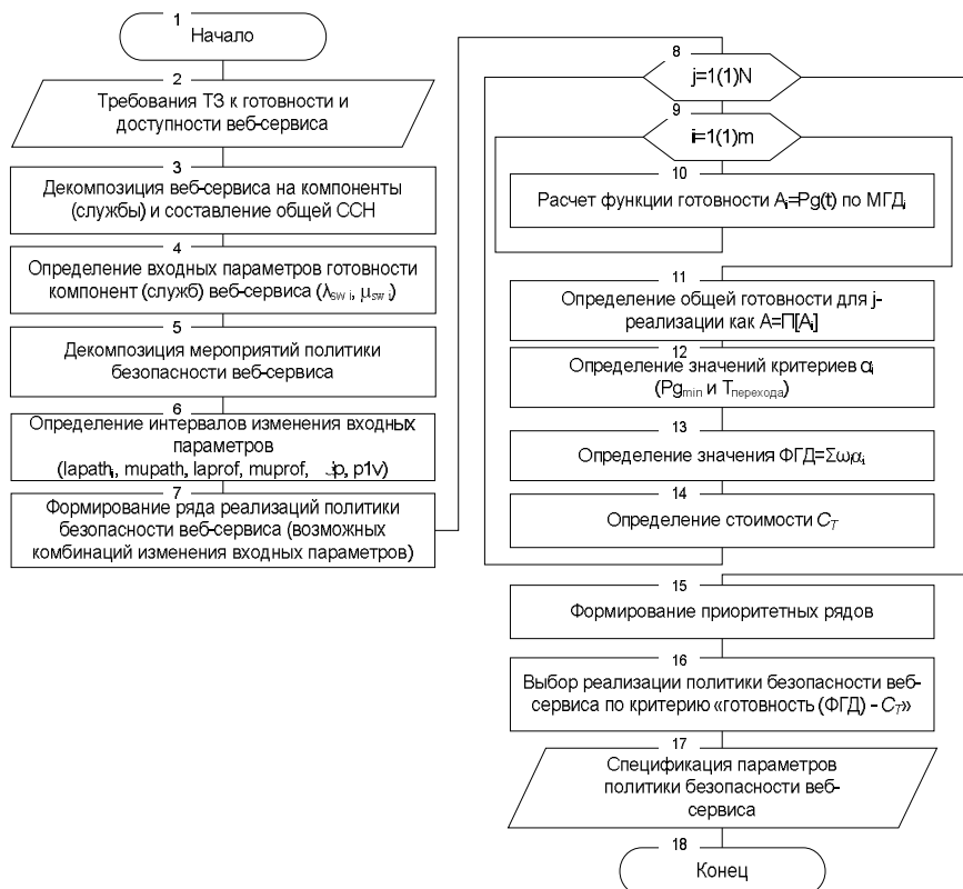
Рис. 2. Метод оптимального варианта реализации политики безопасности веб-сервера в условиях атак на доступность и отказов ПС его компонент
