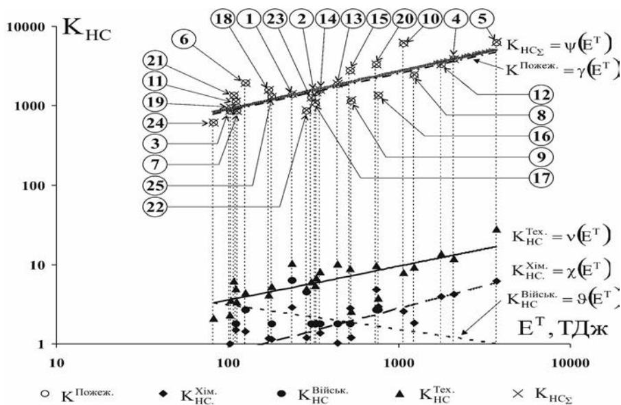
Рис. 5. Графічні залежності між середньодобовою енергією техногенного походження ( E^T ), кількістю надзвичайних ситуацій ( K_{\text{НС}} ) різного походження ( K_{\text{Пожеж.}} – пожежі; K_{\text{Хім.НС}} – надзвичайні ситуації хімічного походження; K_{\text{Військ.НС}} – вибухи боєприпасів; K_{\text{Тех.НС}} – надзвичайні ситуації техногенного походження) та їх сумарною кількістю ( K_{\text{НС}\Sigma} ) в регіонах України (нумерація областей наведена в алфавітному порядку і відповідає рис. 3)
