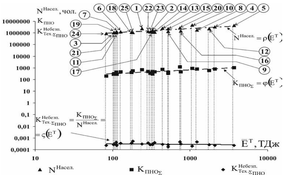
Рис. 4. Графічні залежності між середньодобовою енергією техногенного походження ( E^T ), чисельністю населення ( N^{\text{Насел.}} ), сумарною кількістю потенційно небезпечних об'єктів ( K_{\text{ПНО}\Sigma} ) та показником техногенної безпеки за адитивною кількістю потенційно небезпечних об'єктів на душу населення ( K_{\text{Небезп. Тех.}\Sigma\text{ПНО}} ) в регіонах України (нумерація областей наведена в алфавітному порядку і відповідає рис. 3)
