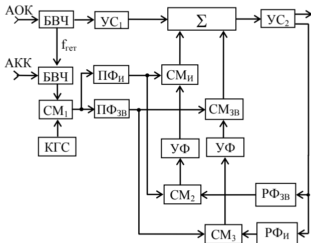
Рис. 1. Общая структура автокомпенсационного устройства
