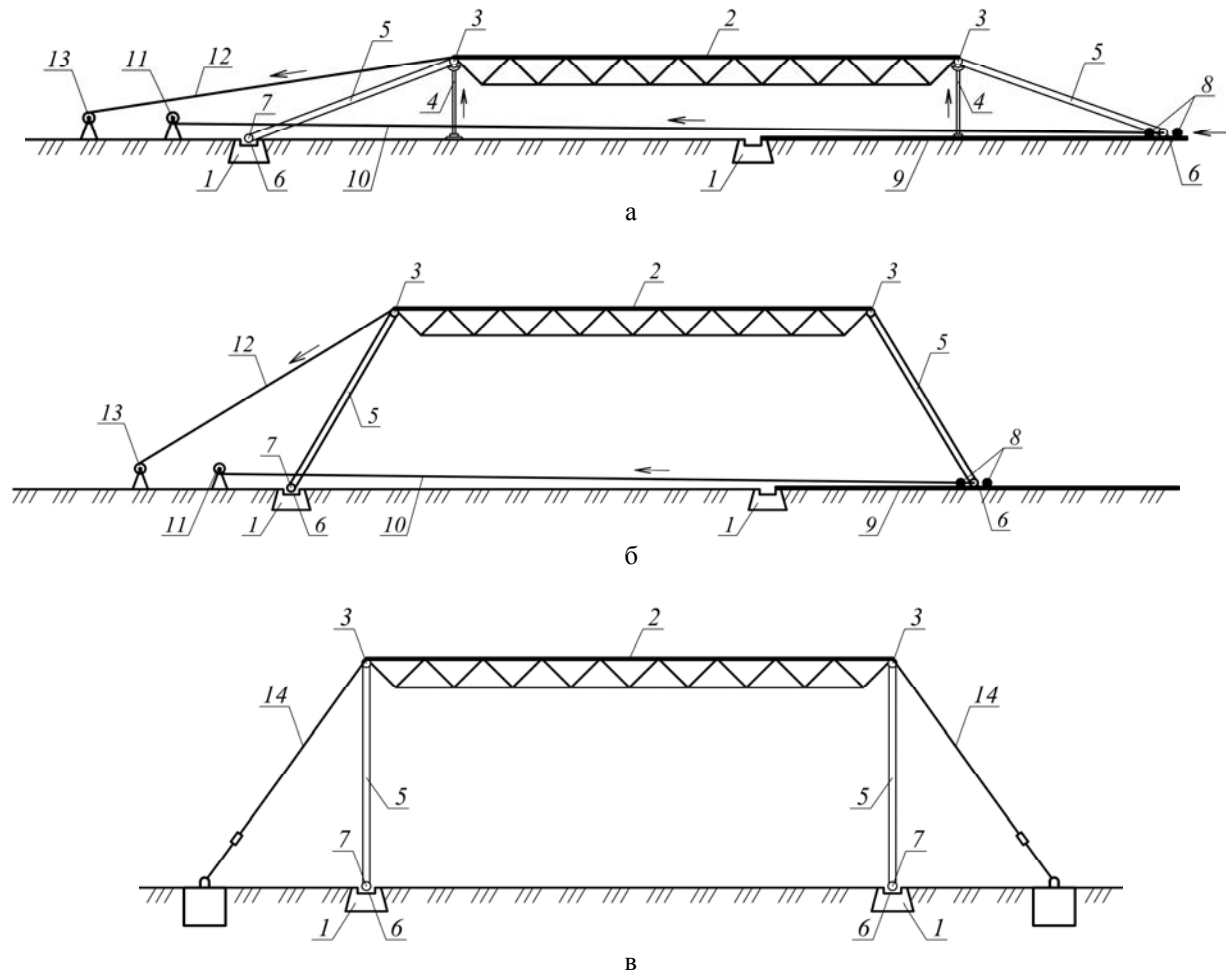
Рис. 2. Технологічні стадії зведення каркасу будівлі із структурно-вантовим сталезалізобетонним покриттям:
