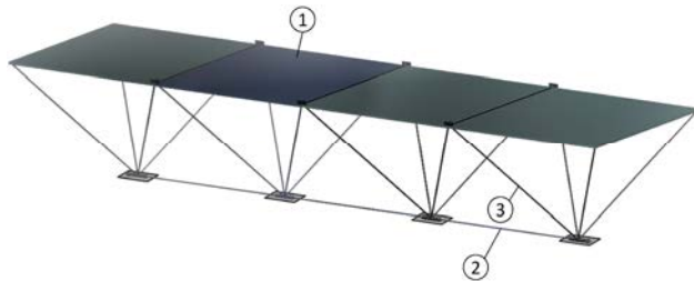
Рис. 1. Лінійний елемент збірного сталезалізобетонного структурно-вантового покриття: 1 – верхній пояс; 2 – нижній пояс; 3 – структурна решітка
