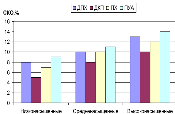
Рис. 3. Среднеквадратическое отклонение ортогональных преобразований при обработке изображений разной степени насыщенности
