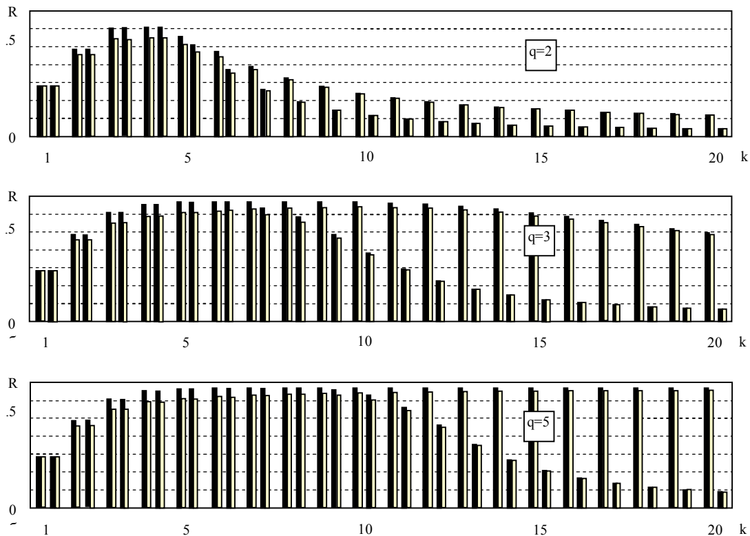
Рис. 1. Залежність пропускної спроможності R від кількості каналів k при декількох відношеннях сигнал/шум q для систем автосупроводження за дальністю (перша пара стовбців) та за радіальною швидкістю (друга пара стовбців):
