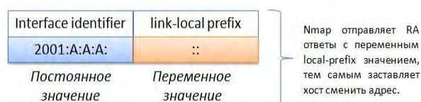
Рис. 8. Принцип работы Nmap скрипта для разведки IPv6 адресов
