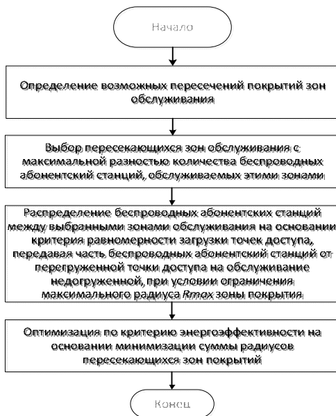
Рис. 4. Алгоритм оптимизации покрытия
