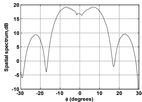
Рис. 1. Реализация СФ (7) для 2 когерентных сигналов с \theta_1 = -4^\circ , \theta_2 = 4.5^\circ
