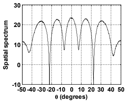
Рис. 2. Реализация СФ (7) для 5 когерентных сигналов, N_{\text{пв}} = 100
