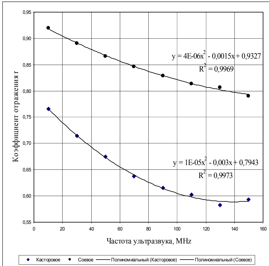
Рис. 1. Частотная зависимость коэффициента отражения
