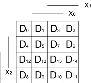
Рис. 4. Карта Карно для ОЛФ типа 4
