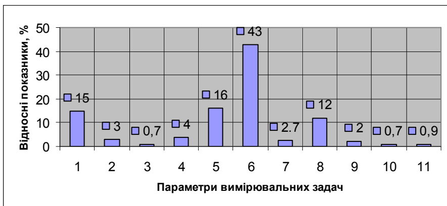
Рис. 1. Відносні показники частоти визначення вимірюваних (контрольованих) параметрів у вимірювальних задачах у ракетному комплексі оперативно-тактичного призначення ( Примітка. Номери вимірювальних (контрольованих) параметрів на вісі абсцис відповідають порядку нумерації рядків в графах „№ з/п” і „Відносне значення” в табл. 2.)
