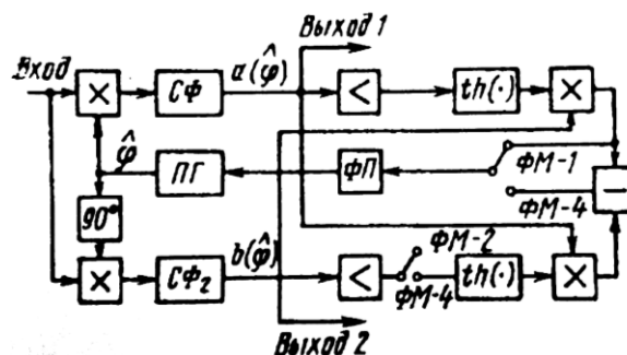
Рис. 1. Оптимальная система восстановления несущей
