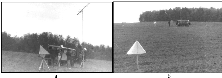
Рис. 1. Ответчики: а – конструкция; б – расположение на местности
