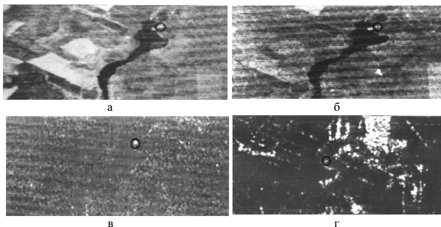
Рис. 2. Фрагмент четырехчастотного радиолокационного изображения полигона в мм (а), см (б), дм (в) и метровом (г) диапазонах
