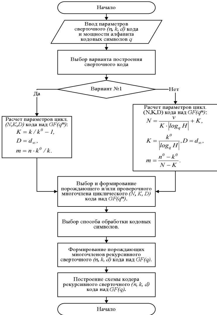
Рис. 1. Схема алгоритма построения рекурсивных сверточных кодов
