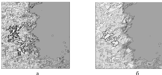
Рис. 5. Поля фрактальных размерностей при s = 9 (а) и s = a = 17 (б)
