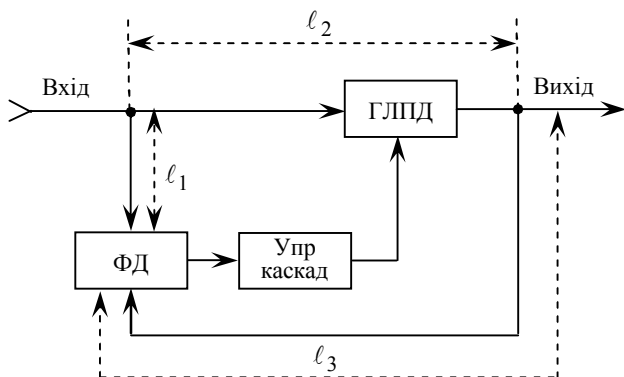
Рис. 1. Ідеалізована система ФАПЧ
