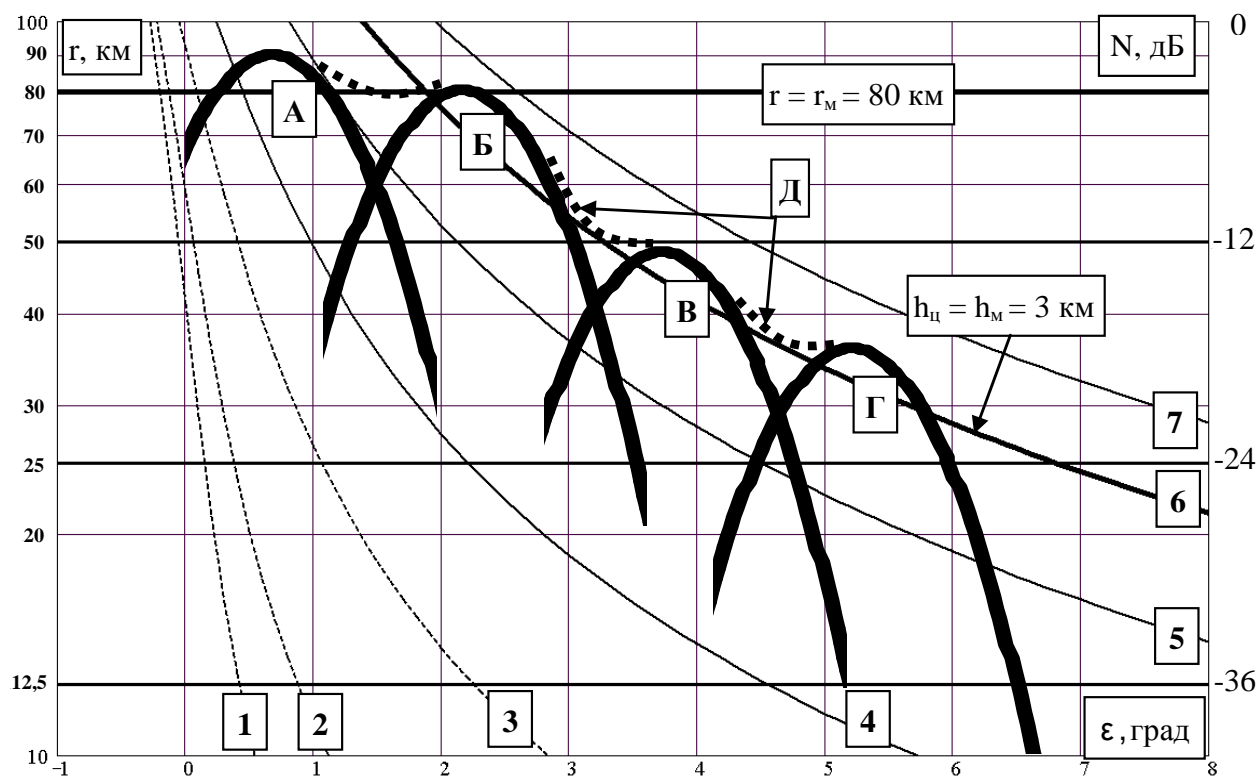
Рис. 4. Вертикальний перетин зони виявлення РЛС в прямокутних координатах \epsilon - r
