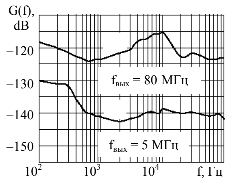
Рис. 11. Распределение фазовых шумов в полосе частот 1 Гц при тактовой частоте 30 МГц и коэффициенте умножения 10
