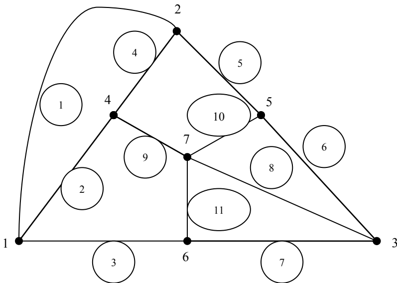
Рис. 1. Граф G(V, E)
