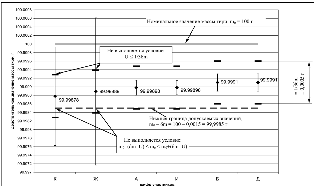
Рис. 1. Данные межлабораторных сличительных калибровок гири с номинальным значением массы 100 г класса точности F_2 и анализ их метрологической правильности
