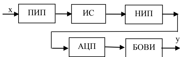
Рис. 1. Функциональная схема ИК
