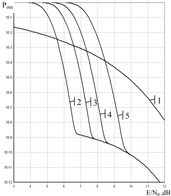
Рис. 2. Зависимости вероятности декодирования кодограмм в каскадных теоретико-кодовых схемах в каналах с группируемыми ошибками
