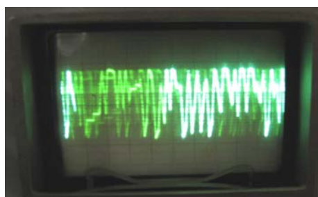
Рис. 3. Временная реализация аналоговой хаотической несущей
