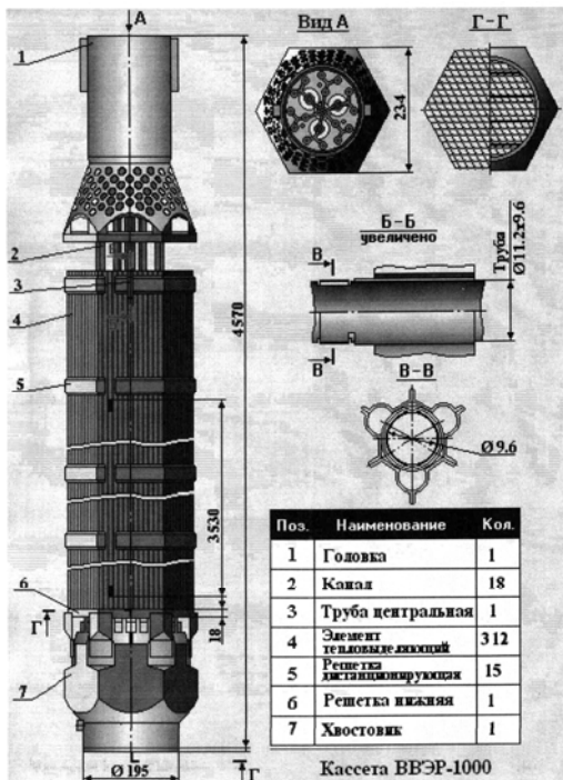
Рис. 5. Кассета ВВЭР-1000
