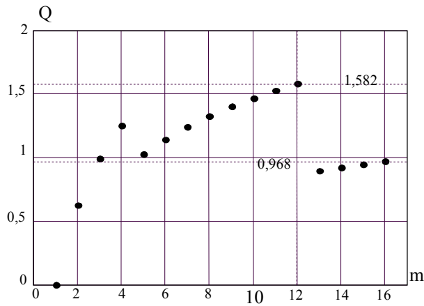
Рис. 1. Графическое решение задачи оптимального усечения ансамбля 2f – 4ф
