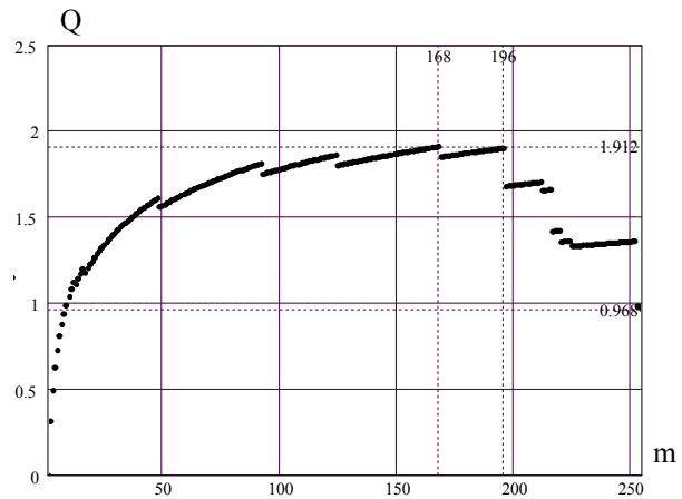
Рис. 2. Графическое решение задачи оптимального усечения ансамбля 4f – 4ф
