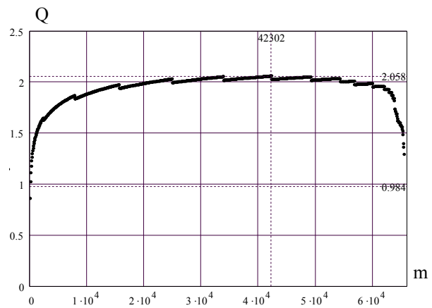
Рис. 3. Графическое решение задачи оптимального усечения ансамбля 8f – 4ф
