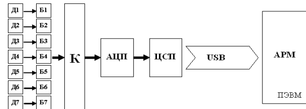
Рис. 4. Схема аппаратно-программного измерительного комплекса: Д – датчик; Б – буферный усилитель; К – коммутатор; АЦП – аналого-цифровой преобразователь; ЦСП – цифровой сигнальный процессор; АРМ – автоматизированное рабочее место
