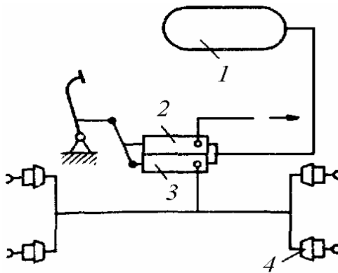
Рис. 2. Схема пневматического привода рабочей тормозной системы автомобиля: 1 – воздушный баллон; 2 – верхняя секция тормозного крана (управления тормозной системой прицепа); 3 – нижняя секция тормозного крана (РТС автомобиля); 4 – тормозные камеры колес
