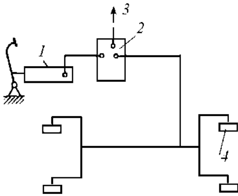
Рис. 1. Тормозная система с гидроприводом и гидровакуумным усилителем: 1 – главный тормозной цилиндр; 2 – гидровакуумный усилитель; 3 – трубопровод к впускному коллектору двигателя; 4 – колесный тормозной цилиндр
