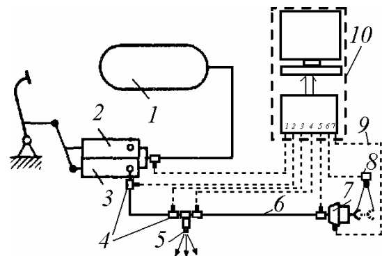
Рис. 3. Схема лабораторной измерительно-экспериментальной установки для исследования пневматического привода рабочей тормозной системы автомобиля:
