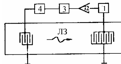
Рис. 2. Генератор с линией задержки на ПЛВ: 1, 4 – согласующие четырехполюсники; 2 – широкополосный усилитель; 3 – частотно-избирательная схема
