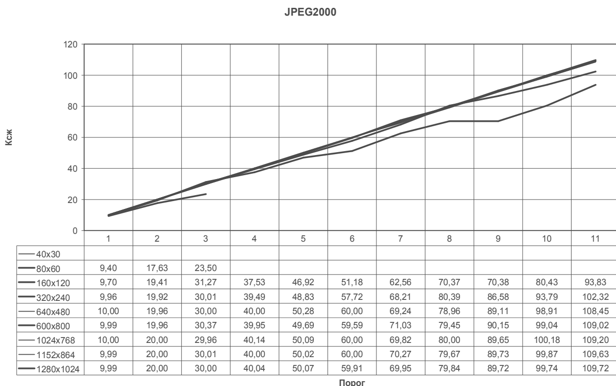
Рис. 2. Зависимость коэффициента сжатия K_{сж} от величины порога фильтрации стандарта JPEG 2000 для изображений разных размеров
