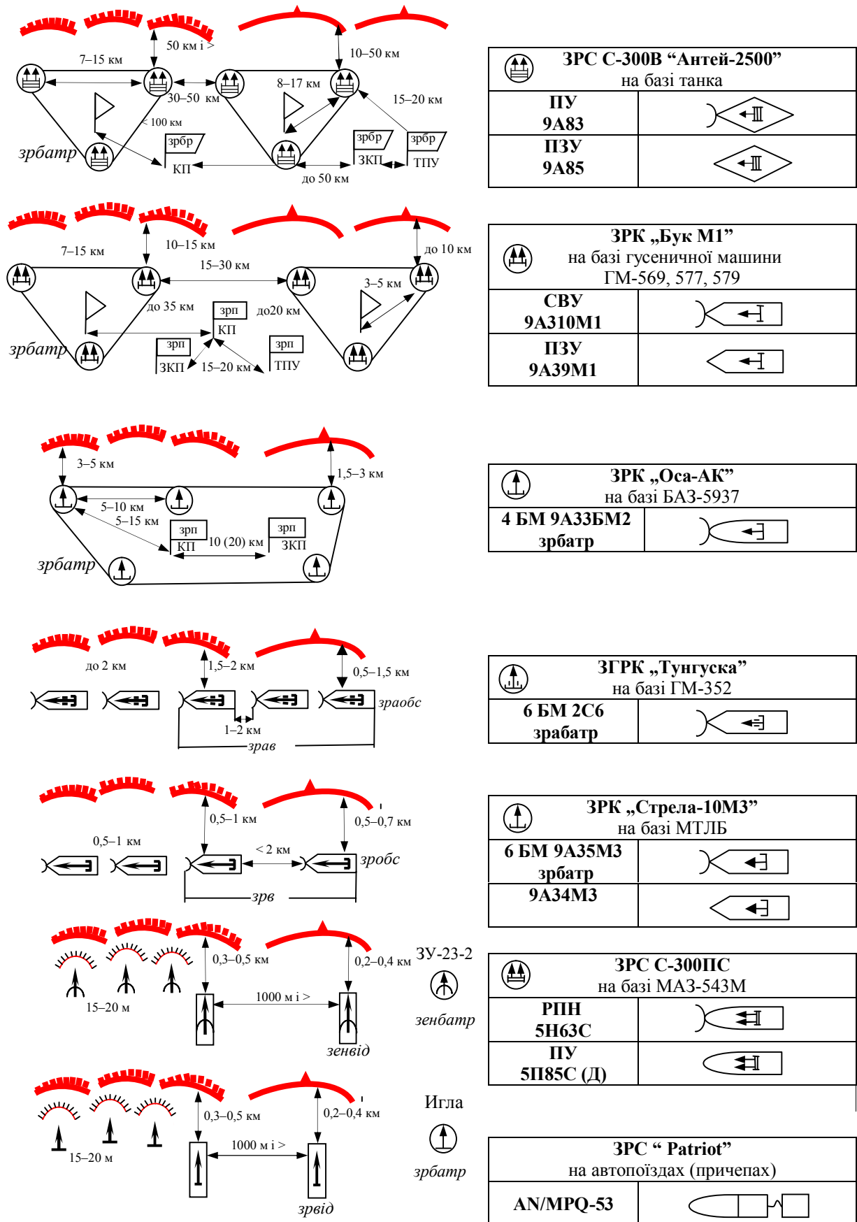
Рис. 1. Умовні позначення в угрупованні ЗРВ
