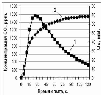
Рис. 7. Характер изменения концентрации CO (ppm) и сигнала ГПИ - U_c (мВ) во времени (с.). T_{\text{пиролиза}}=160 °C: 1 - концентрация CO; 2 - величина U_c . [CO_2]_{\text{max}}=5000 ppm
