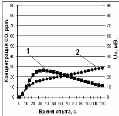
Рис. 2. Характер изменения концентрации CO (ppm) и сигнала ГПИ - U_c (мВ) во времени (с.). T_{\text{пиролиза}}=60 °C: 1 - концентрация CO; 2 - величина U_c . [CO_2]=0
