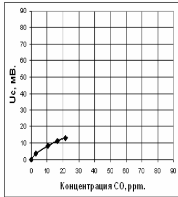
Рис. 3. Зависимость величины сигнала ГПИ - U_c (мВ) от концентрации CO (ppm). T_{\text{пиролиза}}=60 °C; время опыта - 20 с.
