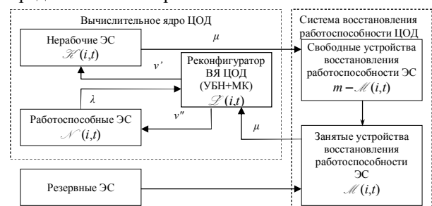
Рис. 2. Обобщенная стохастическая модель функционирования ВЯ ЦОД в ВЭУ
