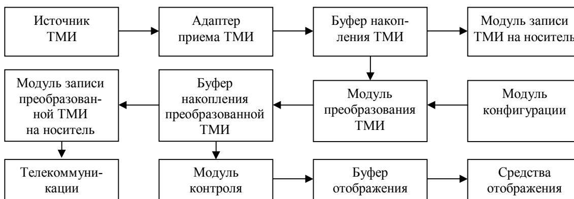
Рис. 2. Схема работы программного обеспечения регистрации и обработки телеметрической информации
