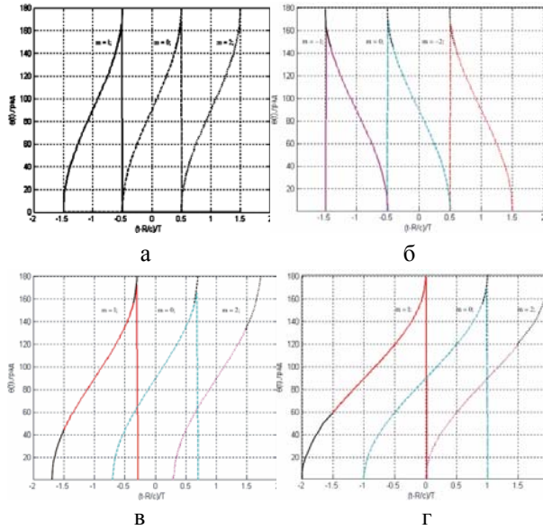
Рис. 3. Характер распределения максимумов ПВС: а – p_n = n ; б – p_n = -n ; в – d\lambda_0^{-1} = 0,7 ; г – d\lambda_0^{-1} = 1
