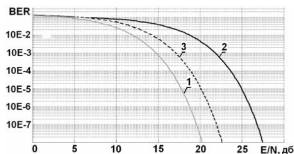
Рис. 1. Залежність BER від ВСШ для QAM-64 у випадках: 1 – теоретична; 2 – без корекції при викривленнях; 3 – з корекцією по п'яти джерелам КС
