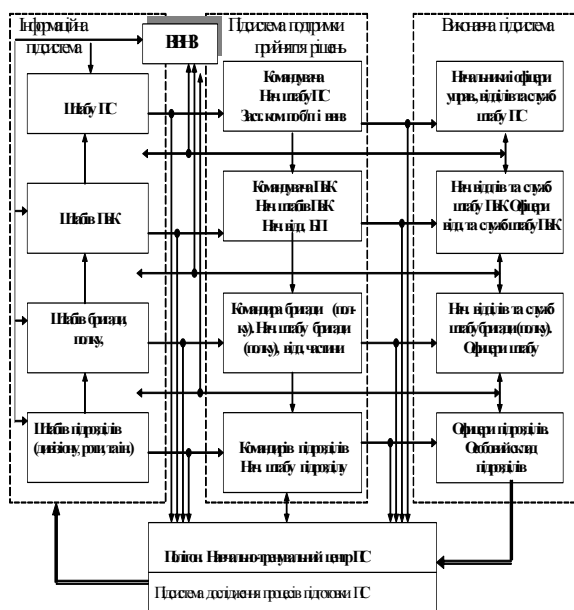
Рис. 1. Організаційно-технічна структура автоматизованої системи управління підготовки РС (функціональний аспект)
