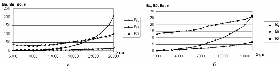
Рис. 8. Расчетные графики изменения характеристик рассеивания Вд, Вб, Вв в зависимости от дальности стрельбы (152-мм СП 2С5; Снаряд ОФ-29: а – заряд Полный; нач. скорость 945 м/с; б – заряд Второй; нач. скорость 560 м/с)
