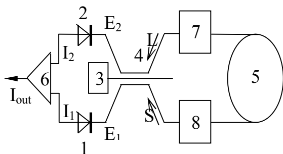
Рис. 1. Схема волоконно-оптичного гіроскопа з відгалуджевачем типу 3×3
