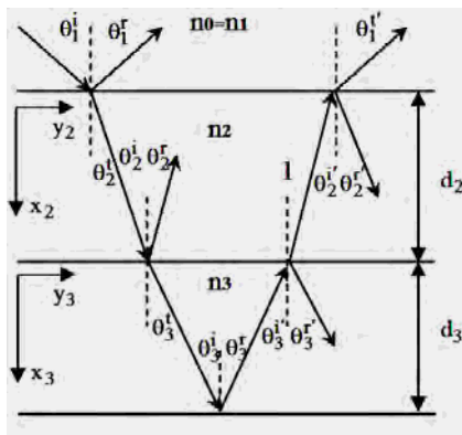
Рис. 6. Распространение электромагнитной волны в N-слоевом покрытии (N=2)
