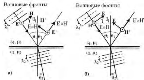
Рис. 2. Распространение плоской ЭМВ через плоскую ПР для ортогональных поляризаций: а – \gamma = 0^\circ , б – \gamma = \pi/2 , рад
