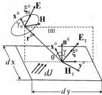
Рис. 1. Пояснение падения ЭМВ с произвольной линейной \gamma \neq 0 и исходной линейной \gamma = 0 поляризациями на элемент dx dy поверхности раздела (ПР)
