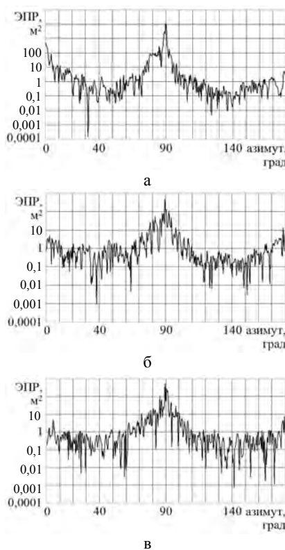
Рис. 4. ДОВИ БПЛА RQ-4B Global Hawk для \lambda=10 см при различных углах места зондирования \epsilon : аа – 0^\circ ; б – 10^\circ ; в – 20^\circ
