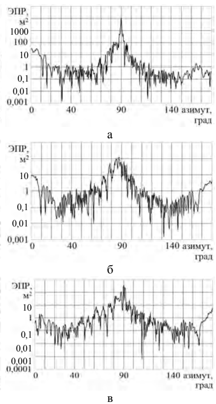
Рис. 5. ДОВИ БПЛА RQ-4B Global Hawk для \lambda=30 см при различных углах места зондирования \epsilon : а – 0^\circ ; б – 10^\circ ; в – 20^\circ
