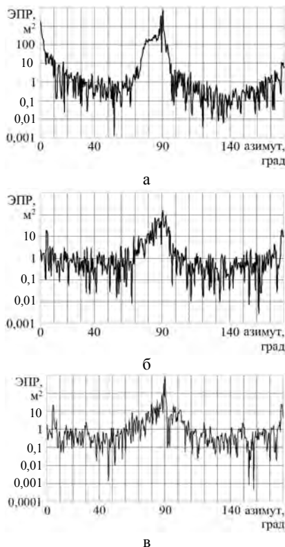
Рис. 3. ДОВИ БПЛА RQ-4B Global Hawk для \lambda=3 см при различных углах места зондирования \epsilon : а – 0^\circ ; б – 10^\circ ; в – 20^\circ
