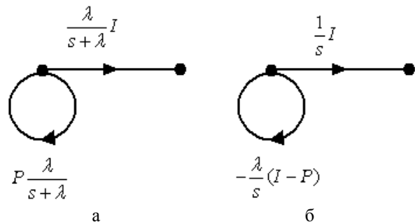
Рис. 3. Матричные графы состояний непрерывного полумарковского процесса
