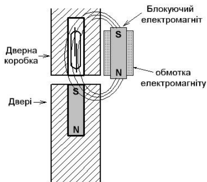
Рис. 3. Нейтралізація герконового датчику за допомогою електромагніту
